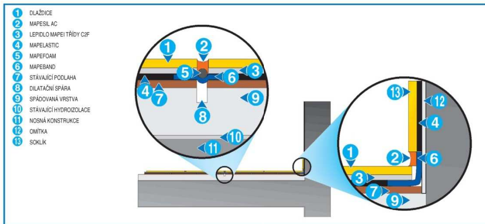
Stavební detail: vodotěsná úprava dilatační spáry
