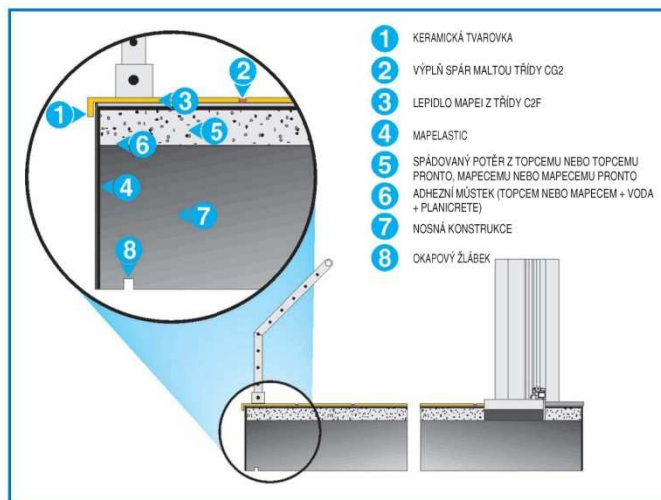
Stavební detail: hydroizolace čelní hrany balkonu
