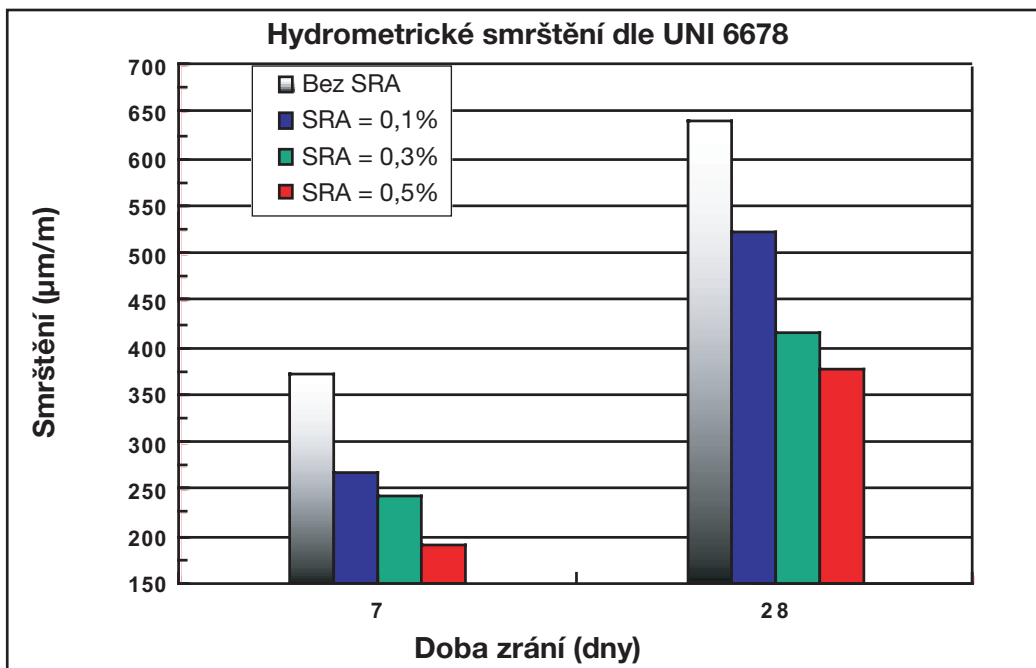
OBR.1 - Hodnoty dosažené s použitím malty obsahující cement CEM I 52,5 R, normový písek a vodu, dle složení navrženého v normě EN 196-1
